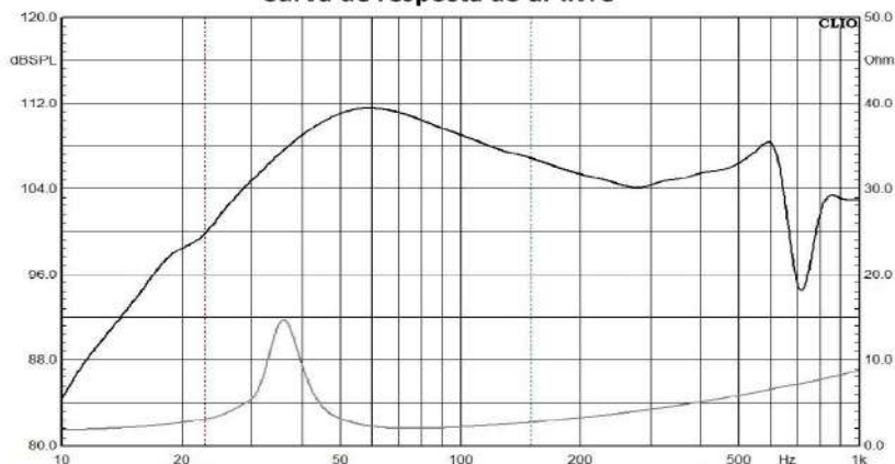
Curva de resposta ao ar livre
