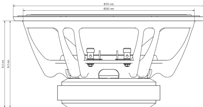
DIMENSIONES EN mm
