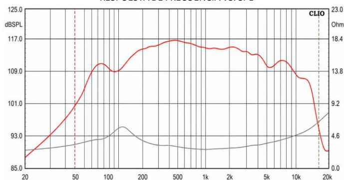
RESPUESTA DE FRECUENCIA VS. SPL
