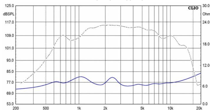
IMPEDANCIA VS. FRECUENCIA
