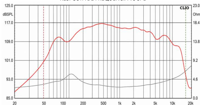
RESPOSTA DE FREQUÊNCIA VS SPL
