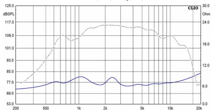
IMPEDÂNCIA VS FREQUÊNCIA
